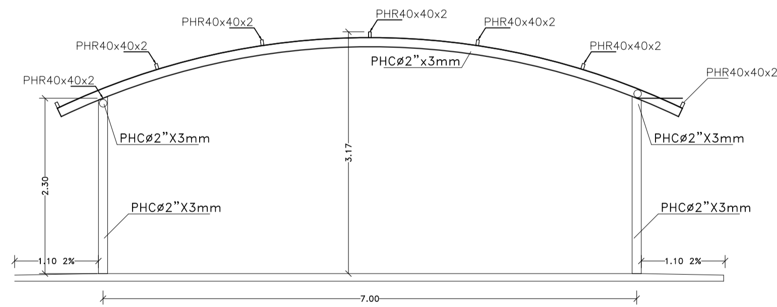
ALZADO INVERNADERO ESC: 1-75
